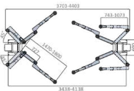
E25 Type M Arms
